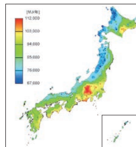
日本各地の太陽光発電量の分布
