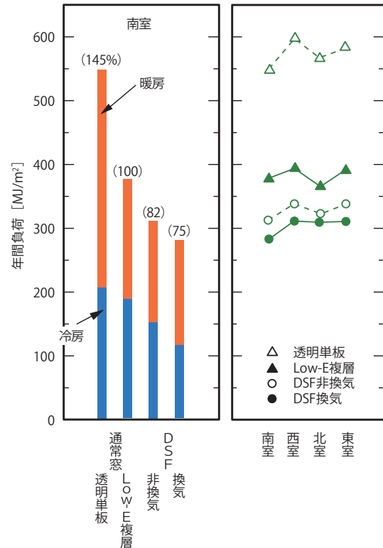
●図2.5b 札幌のペリメータゾーン年間負荷(郡)
