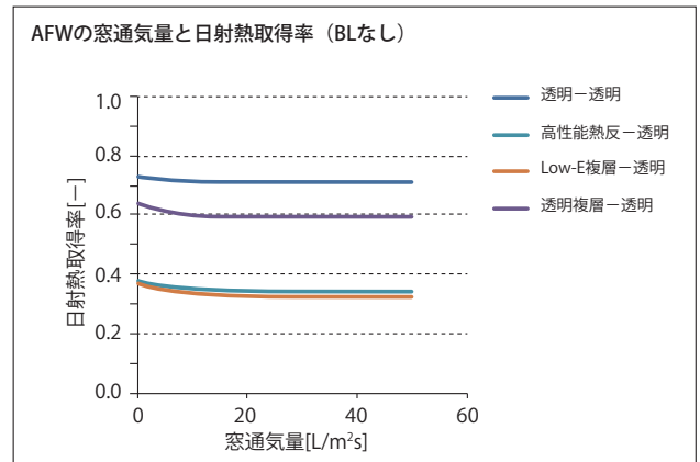
d) 日射熱取得率 (ブラインドなし)
