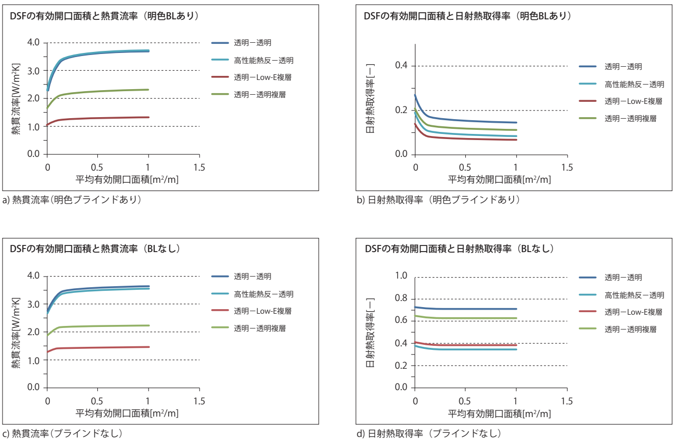
● 図2.3 DSFの窓通気量による熱性能の変化
