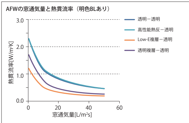
a) 熱貫流率 (明色ブラインドあり)
