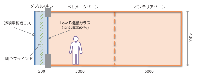
●図2.6 計算モデル断面図
