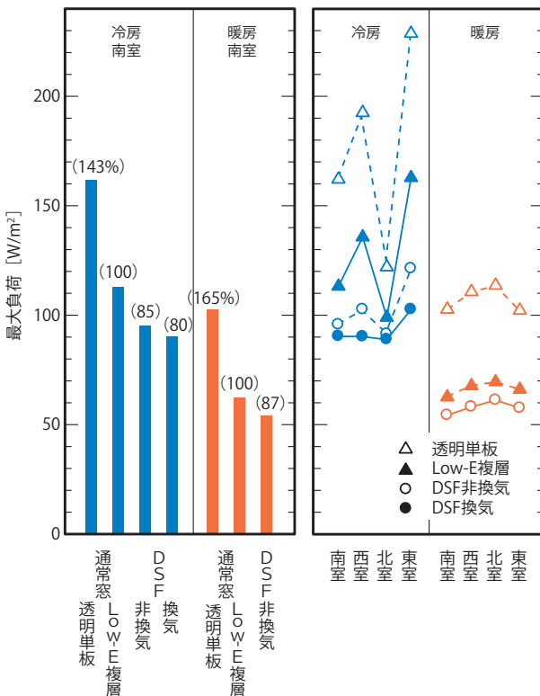
●図2.4a 東京のペリメータゾーン最大負荷(郡)
