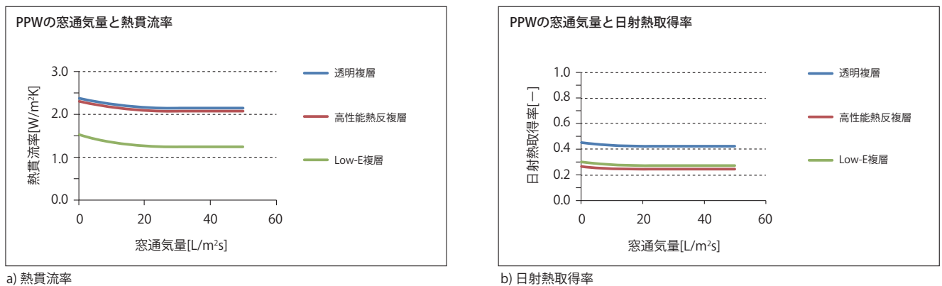
● 図2.1 PPWの窓通気量による熱性能の変化
