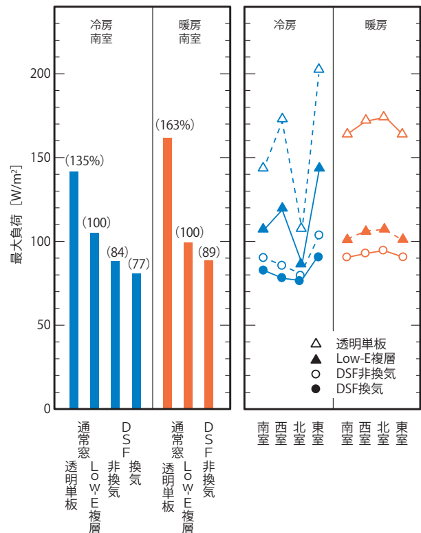
●図2.4b 札幌のペリメータゾーン最大負荷(郡)
