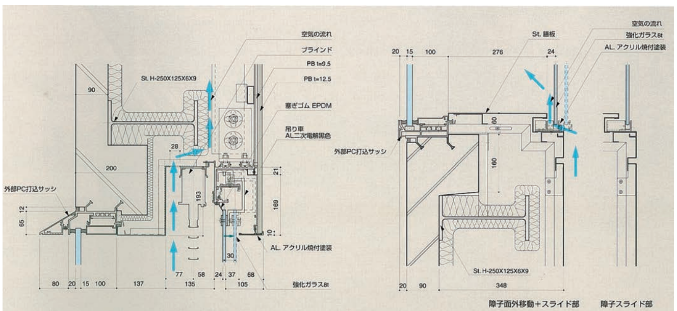
エアフローウィンドウ上部縦断面図
