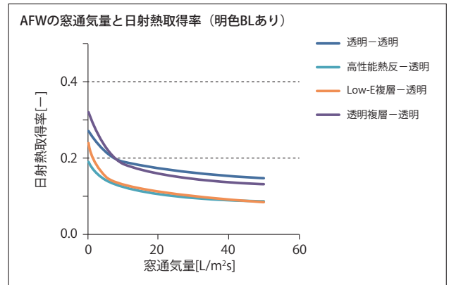
b) 日射熱取得率 (明色ブラインドあり)
