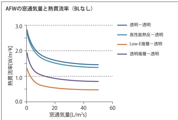
c) 熱貫流率 (ブラインドなし)
